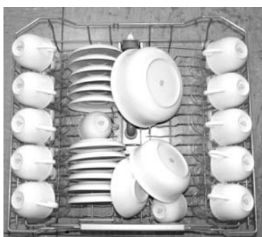
Укладка посуды в верхней корзине
