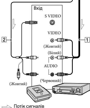
Потік сигналів
