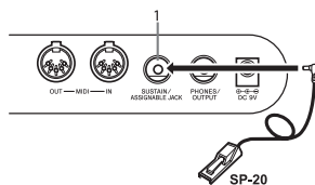
1 Разъем «SUSTAIN/ASSIGNABLE JACK»
